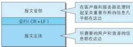
图：HTTP 报文的结构
