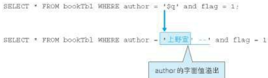
图：SQL 注入攻击的原理
