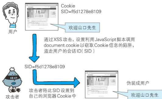
图：会话劫持攻击案例
