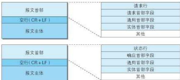
图：请求报文（上）和响应报文（下）的结构
