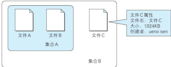
图：WebDAV 扩展的概念
