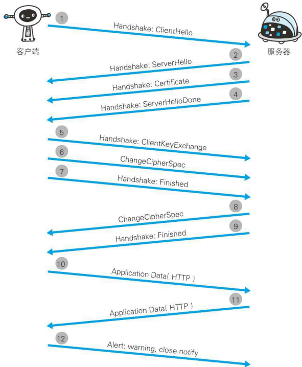
图：HTTPS 通信
