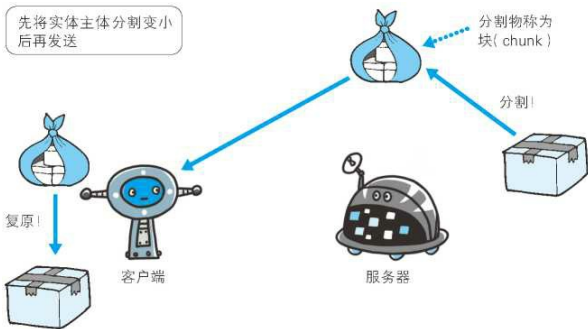
图：分块传输编码
