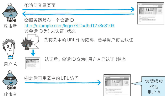
图：会话固定攻击案例
