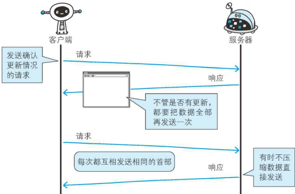
图：以前的 HTTP 通信
