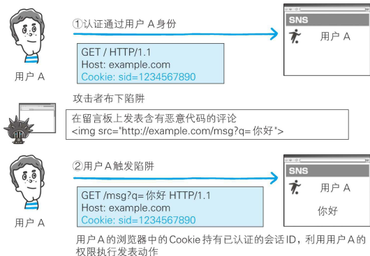
图：跨站点请求伪造的攻击案例
