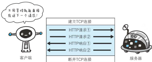
图：不等待响应，直接发送下一个请求
