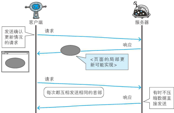
图：Ajax 通信
