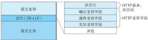
图：响应报文
