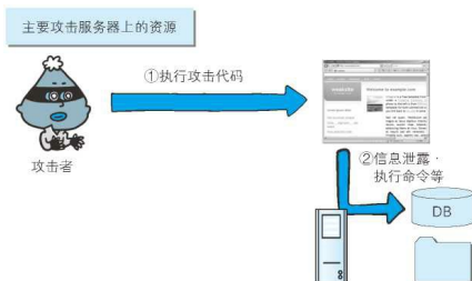
图：主动攻击
