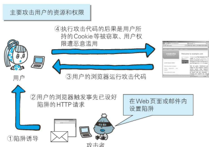
图：被动攻击
