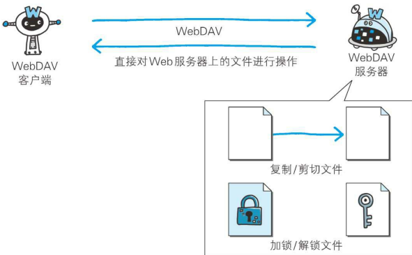
图：WebDAV
