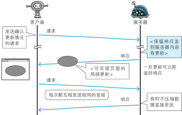
图：Comet 通信
