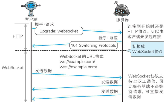
图：WebSocket 通信
