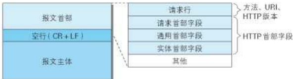
图：请求报文
